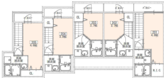
3階平面図
