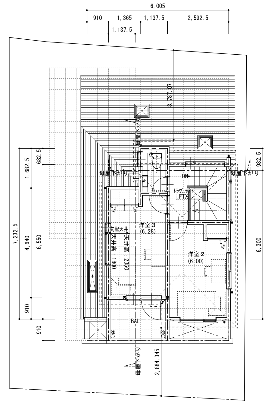
3階平面図 1:100
