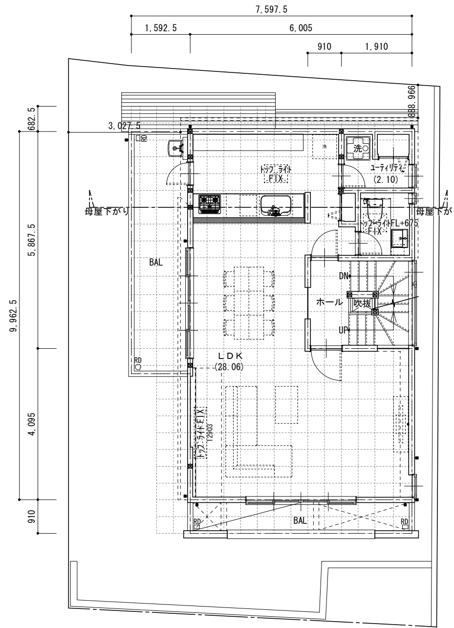
2階平面図 1:100
